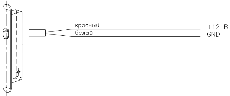
Рис.2. Подключение eld.l-03.nc.C11.40.3.0.dc.00
